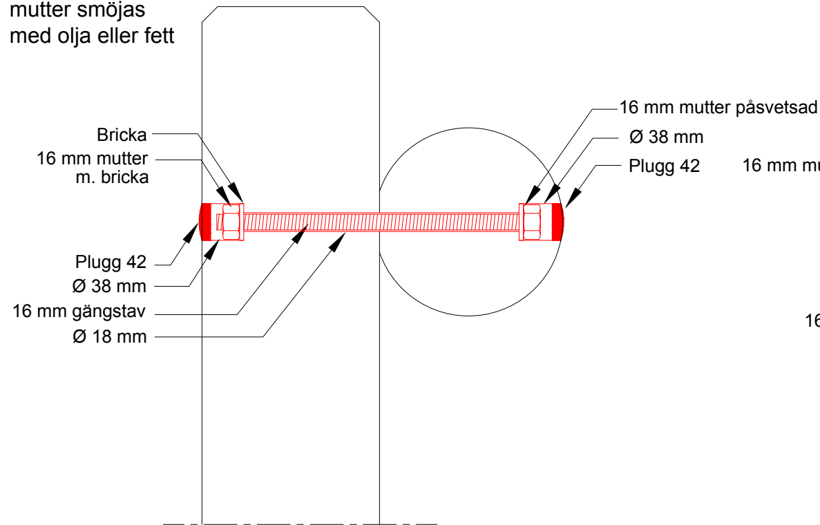
2A: Sidomontering utan distansstycke
