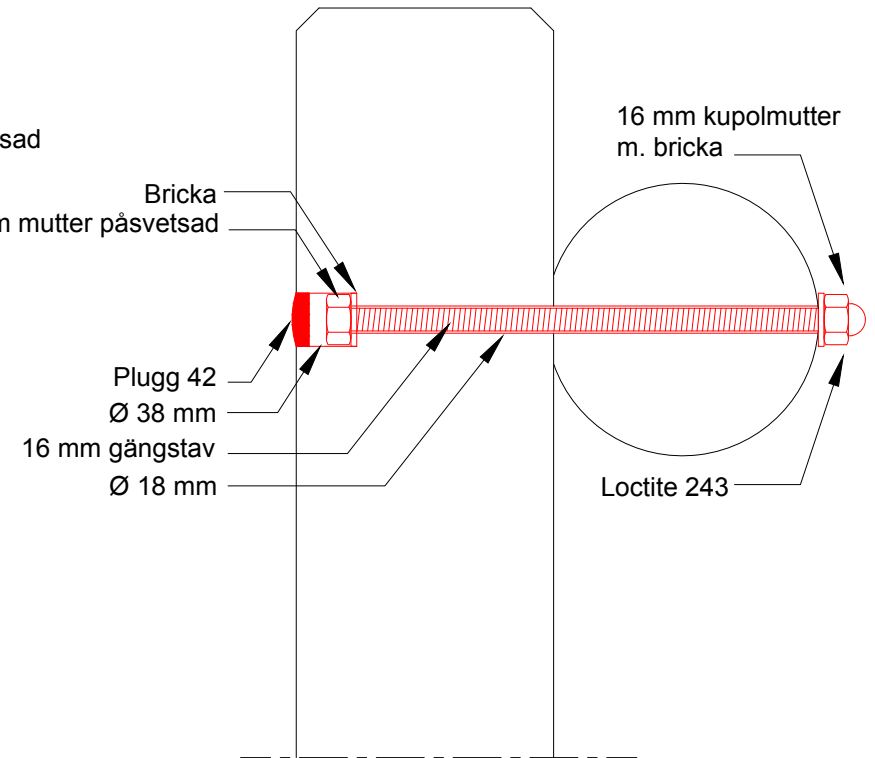
2B: Sidomontering utan distansstycke - med kupolmutter
